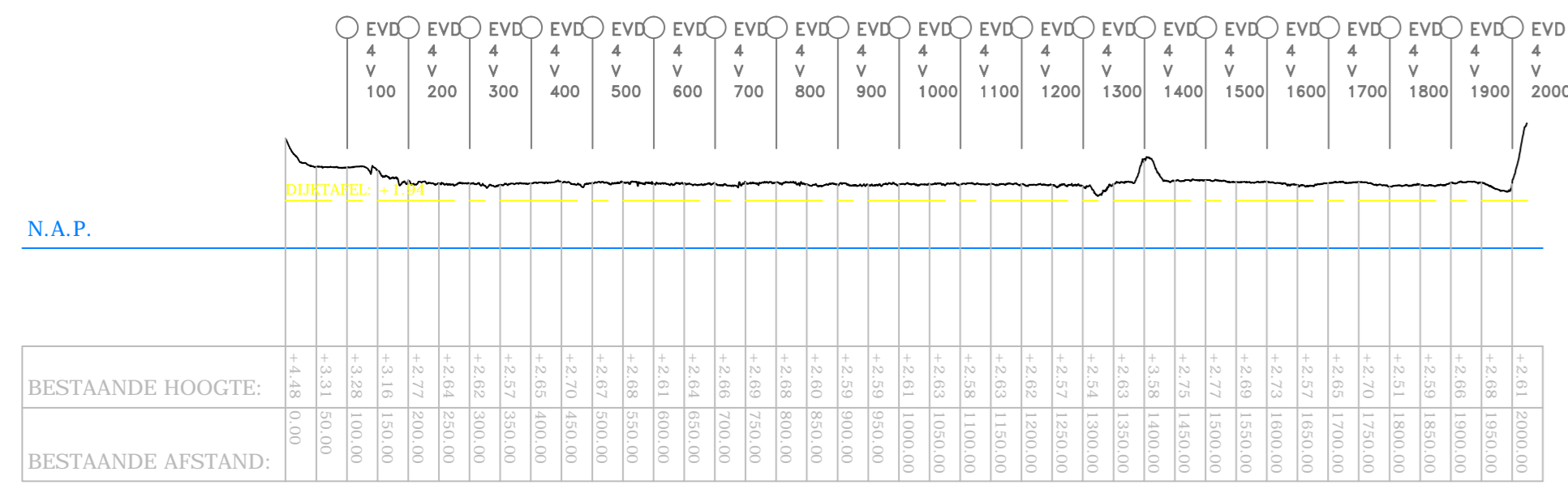
Dijkvak: EVD-4
